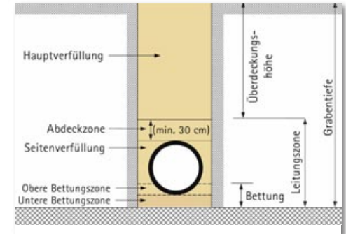
Bild 35: Leitungsgraben in Anlehnung an DIN EN 1610 „Einbau und Prüfung von Abwasserleitungen und -kanälen“
