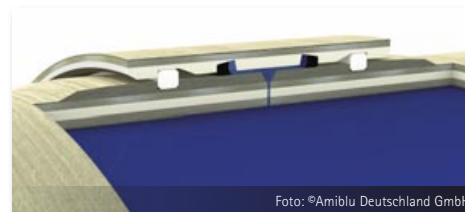
Bild 10: GFK-Rohr mit Scherstabkupplung
