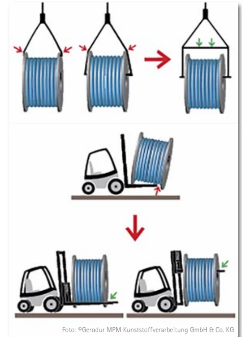
Bild 18: Schäden vermeiden: Entladen und Transportieren von Trommeln
