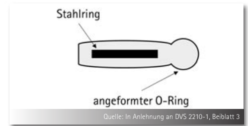
Bild 33: Querschnitt einer Profildichtung mit einvulkanisiertem Stahlring und angeformtem O-Ring
