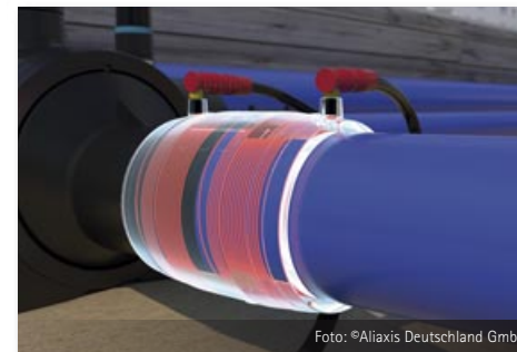
Bild 26: Verfahren: Heizwendel-Schweißen
