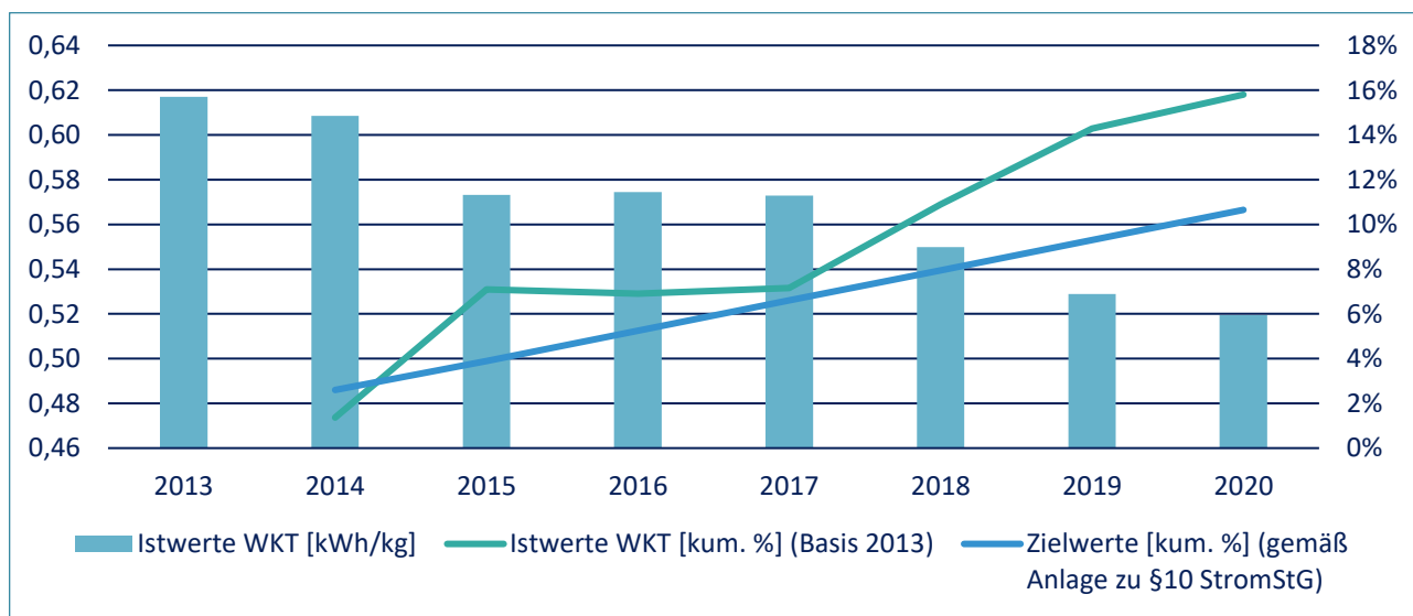
Abbildung 6: Energieeffizienzentwicklung prozentual zum Basisjahr 2013 und absolut
